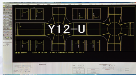
ネスティング図
