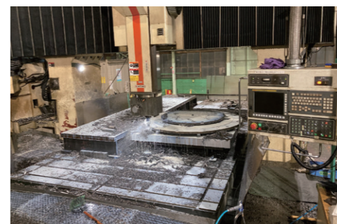
▲切削・フライス (免震フランジ)
