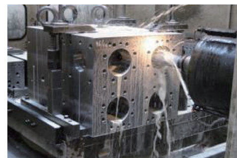
▲大型五面加工機 (マニホールドブロック)
