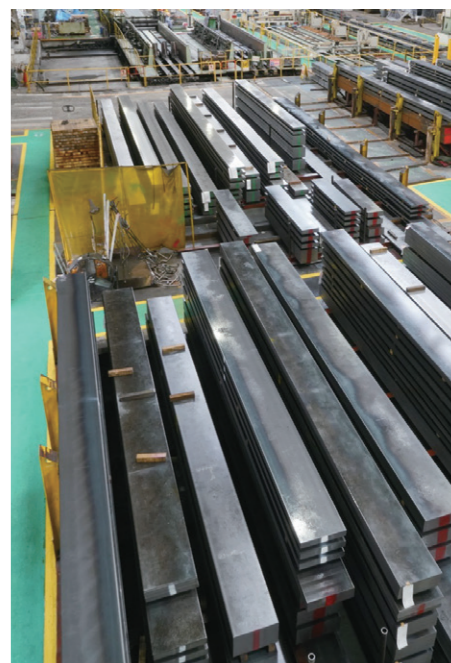
▲スリット製品ヤード
