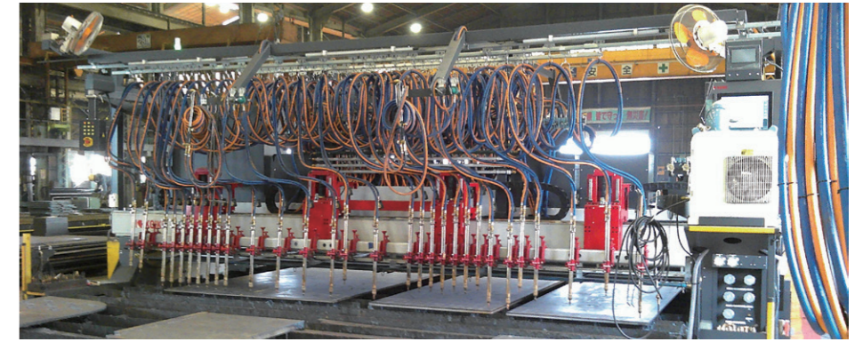
▲フレームブレンダーガス切断機
