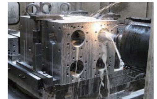
▲大型五面加工機 (マニホールドブロック)
