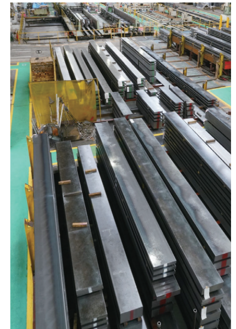
▲スリット製品ヤード
