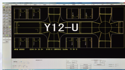
ネステイング図
